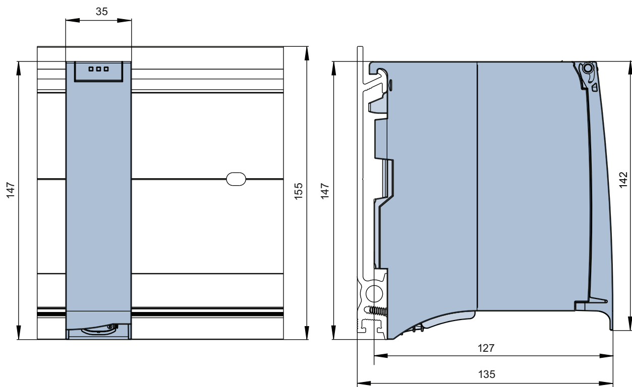
图 A-1 CM PtP RS232 BA 通信模块的尺寸图
