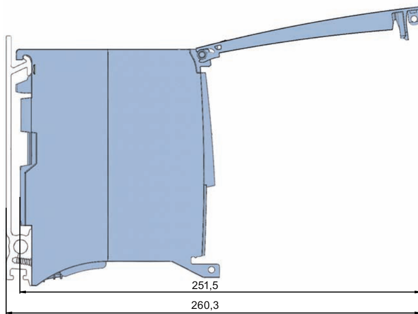
图 A-2 带开放式前面板的 CM PtP RS232 BA 通信模块的尺寸图
